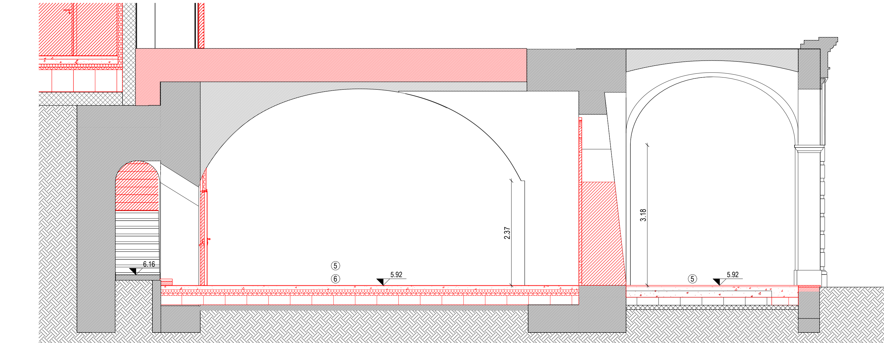
2) sezione AA - costruzioni
