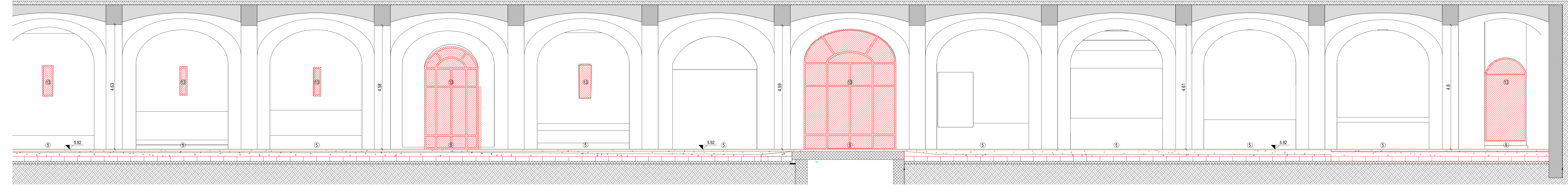
5b) sezione DD - costruzioni - vista 2
