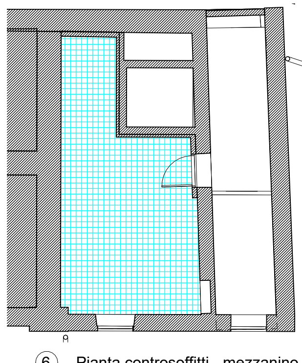
6 Pianta controsoffitti - mezzanino 1 : 100
