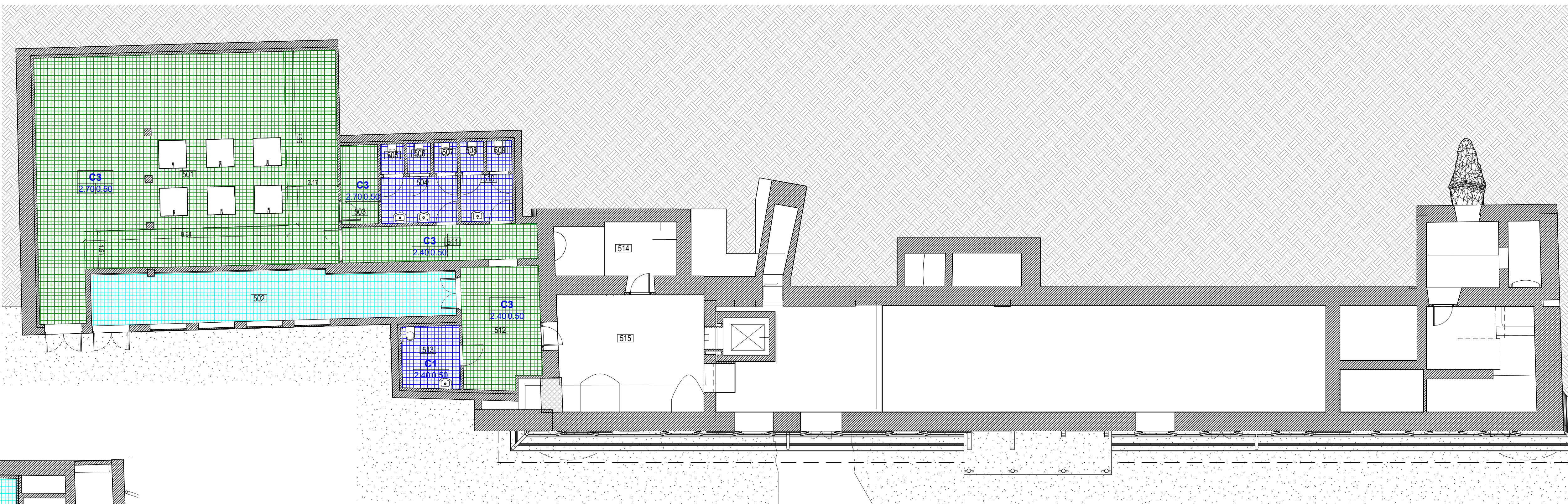
3 Pianta controsoffitti - primo seminterrato - VA 1 : 100
