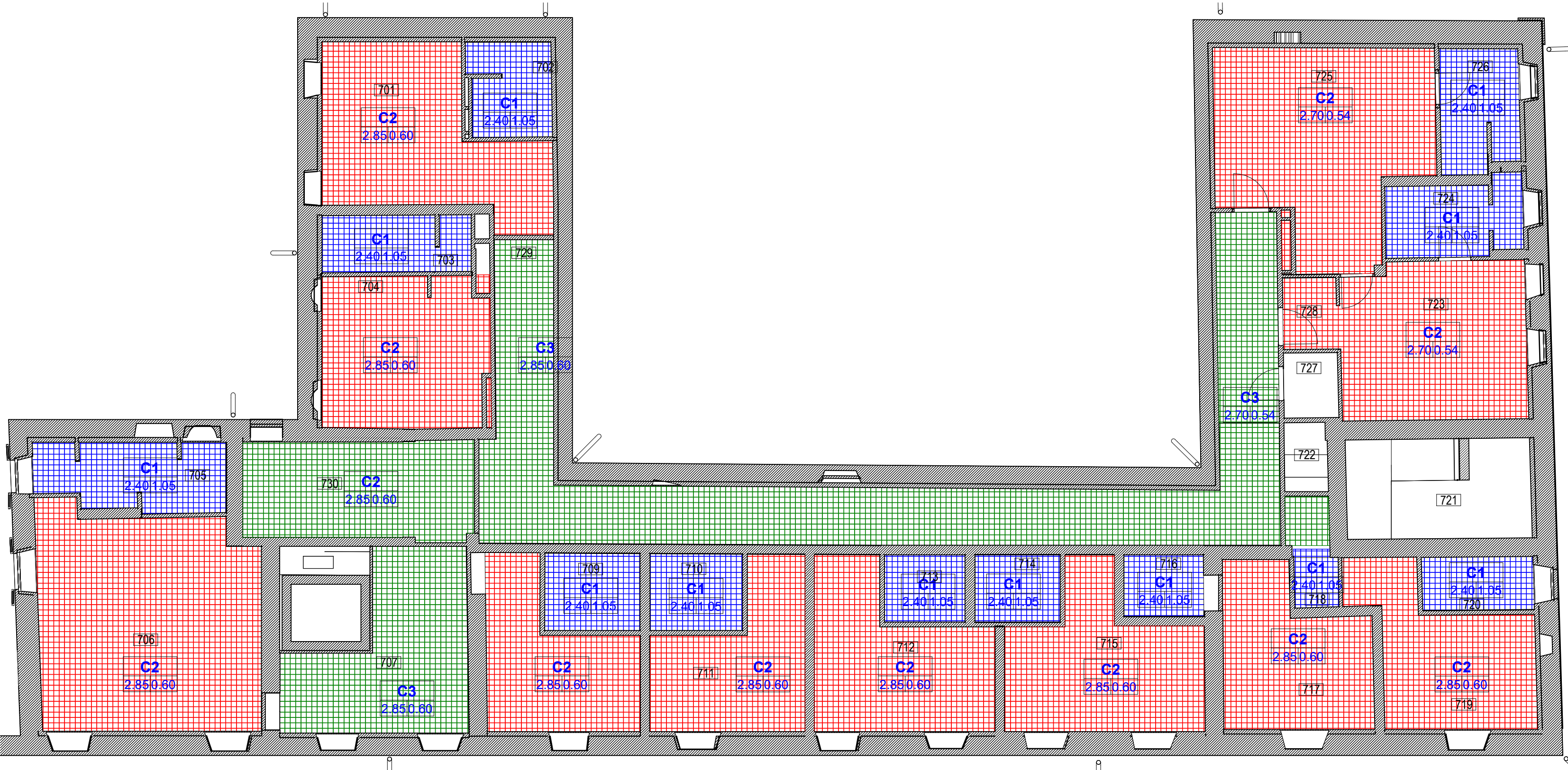
1 Pianta controsoffitti - primo piano - VA 1 : 100
