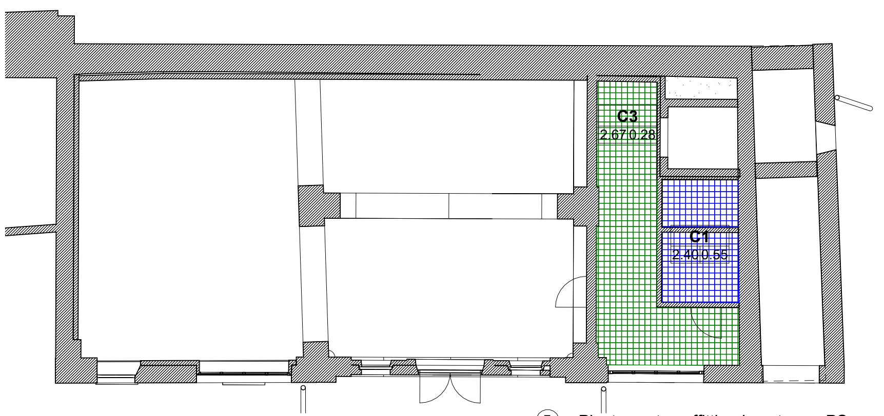
5 Pianta controsoffitti - piano terra - PS 1 : 100
