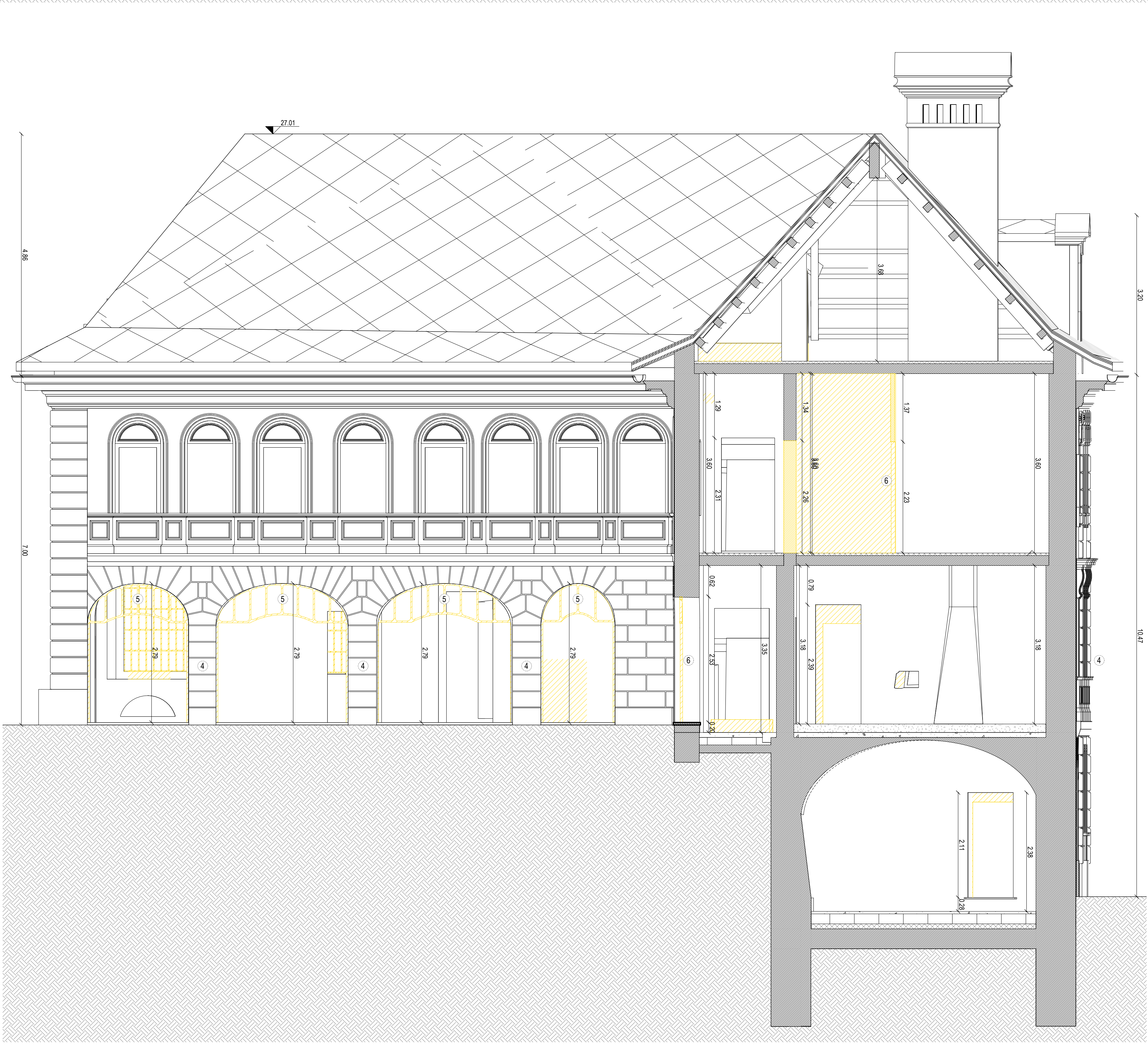
2 sezione LL - demolizioni
