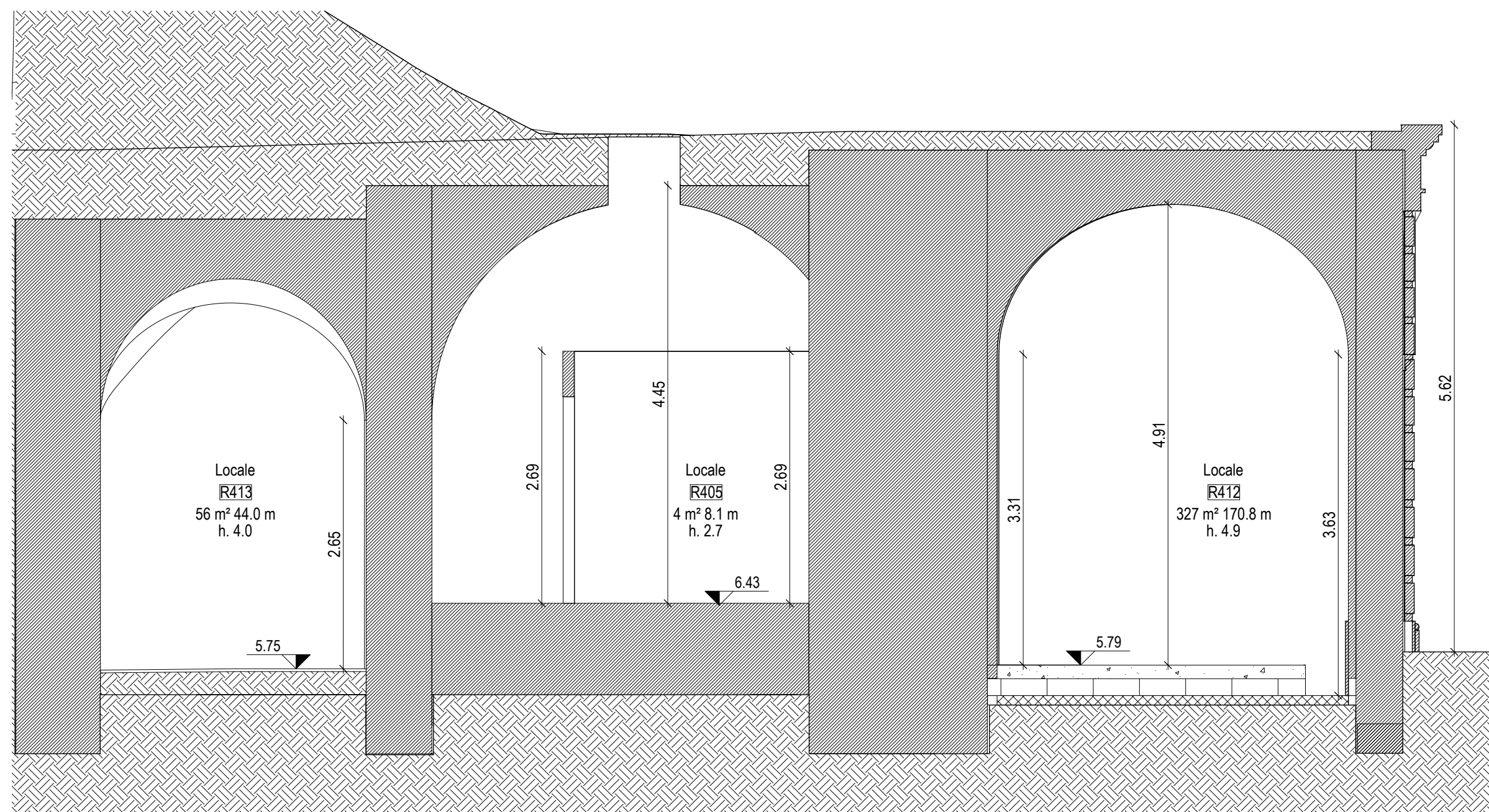
4 sezione CC - rilievo
