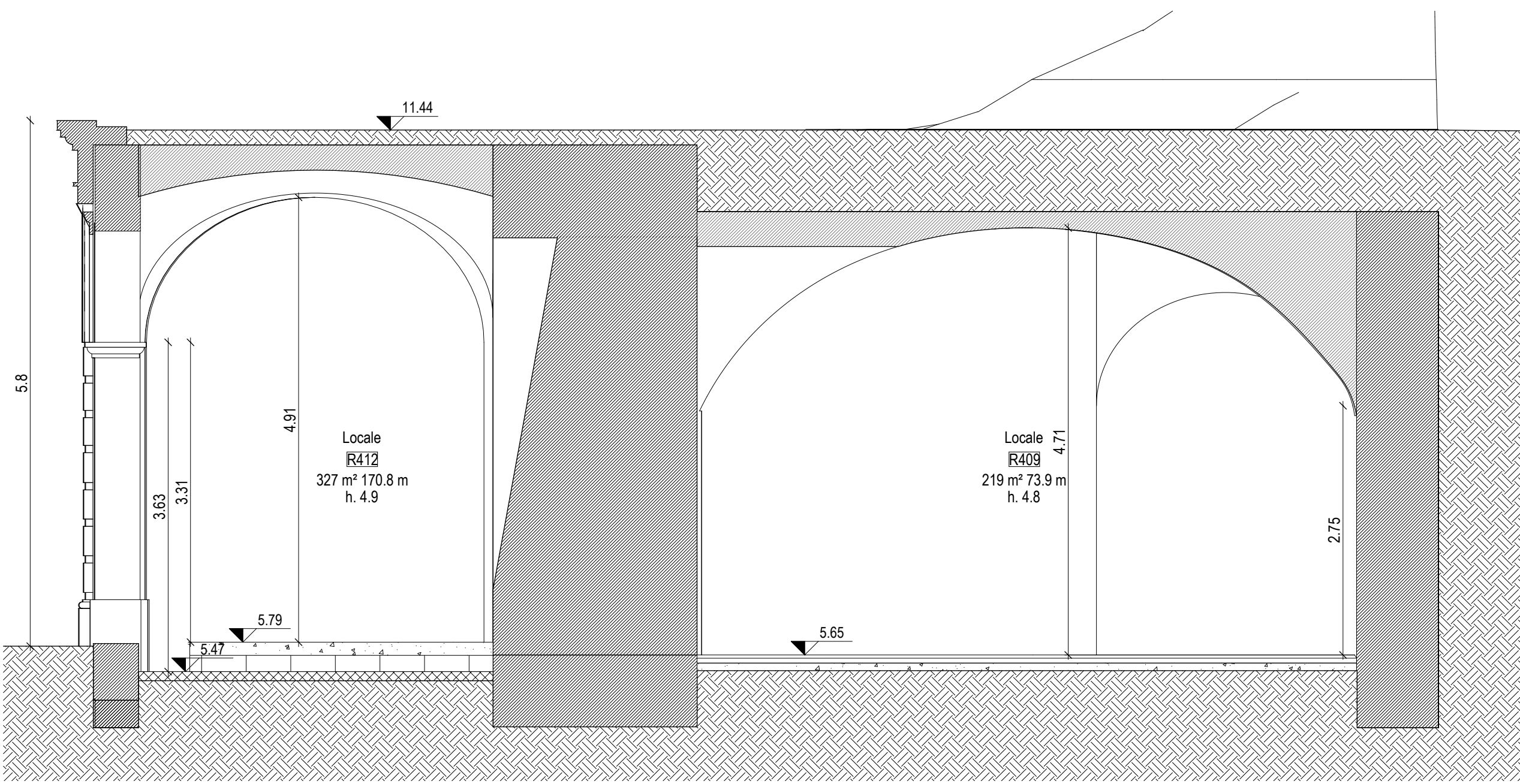
3 sezione BB - rilievo
