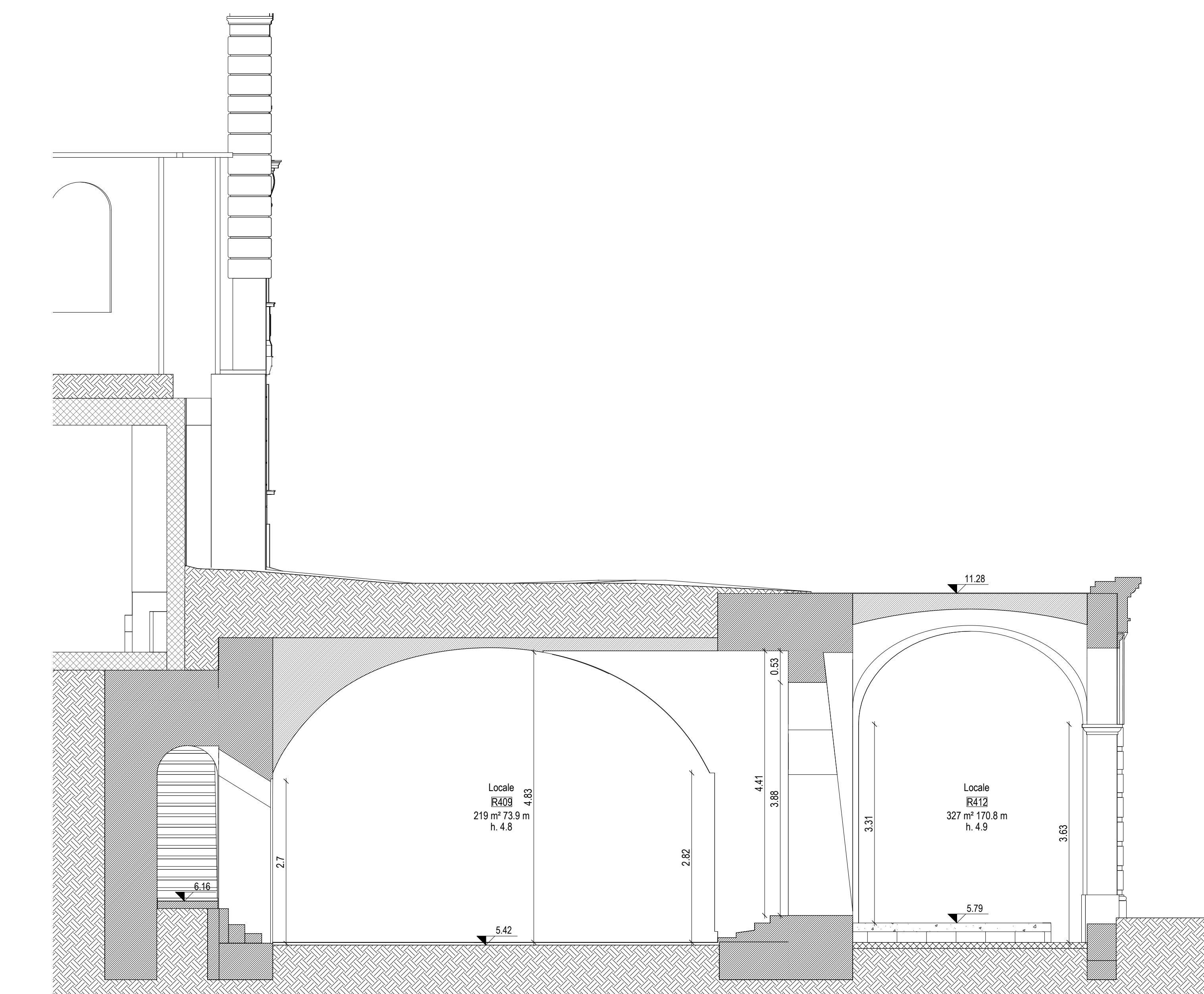
2 sezione AA - rilievo
