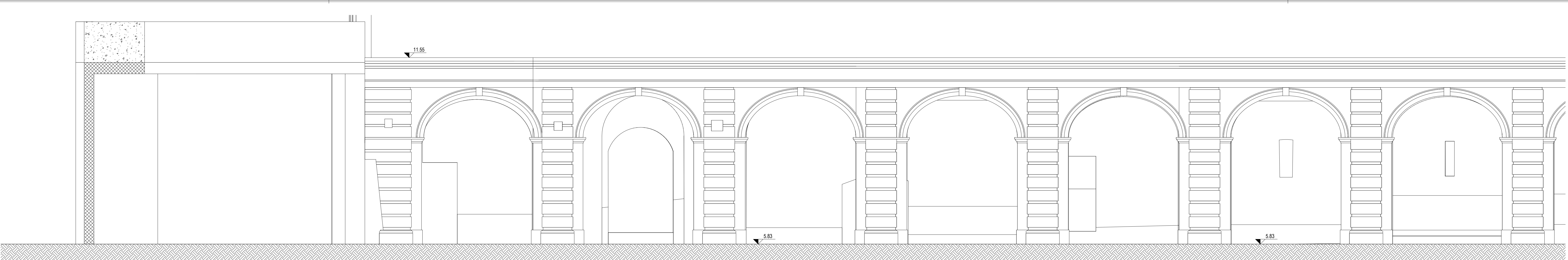
1a prospetto SUD - rilievo - vista 1
