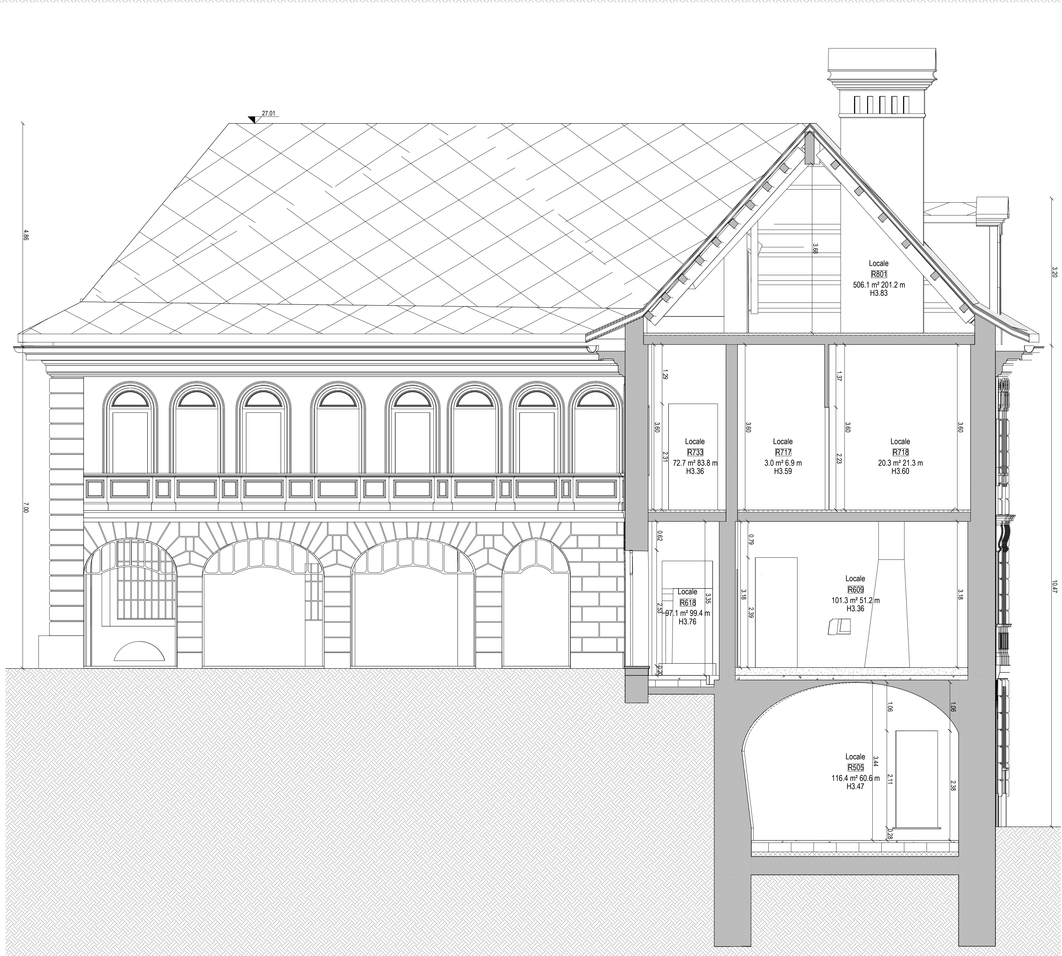
② sezione LL - rilievo
