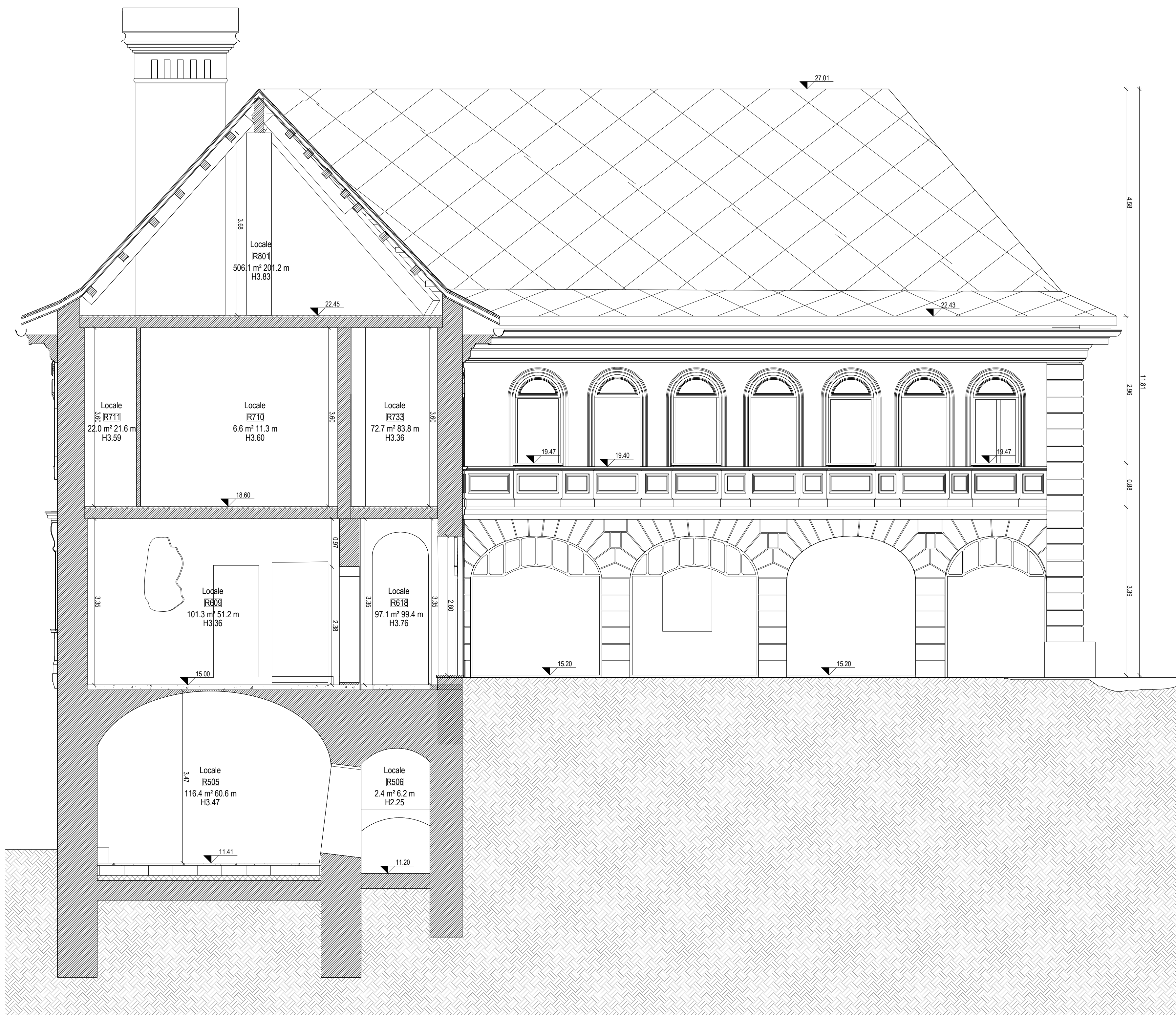
2 sezione GG - rilievo
