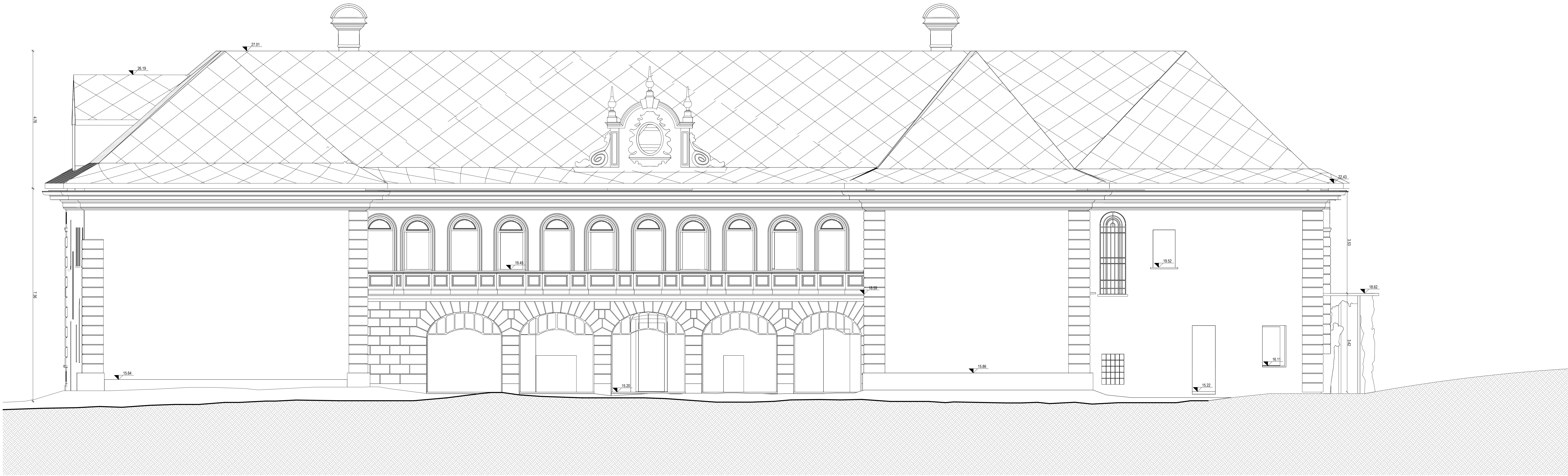
3 prospetto NORD - rilievo
