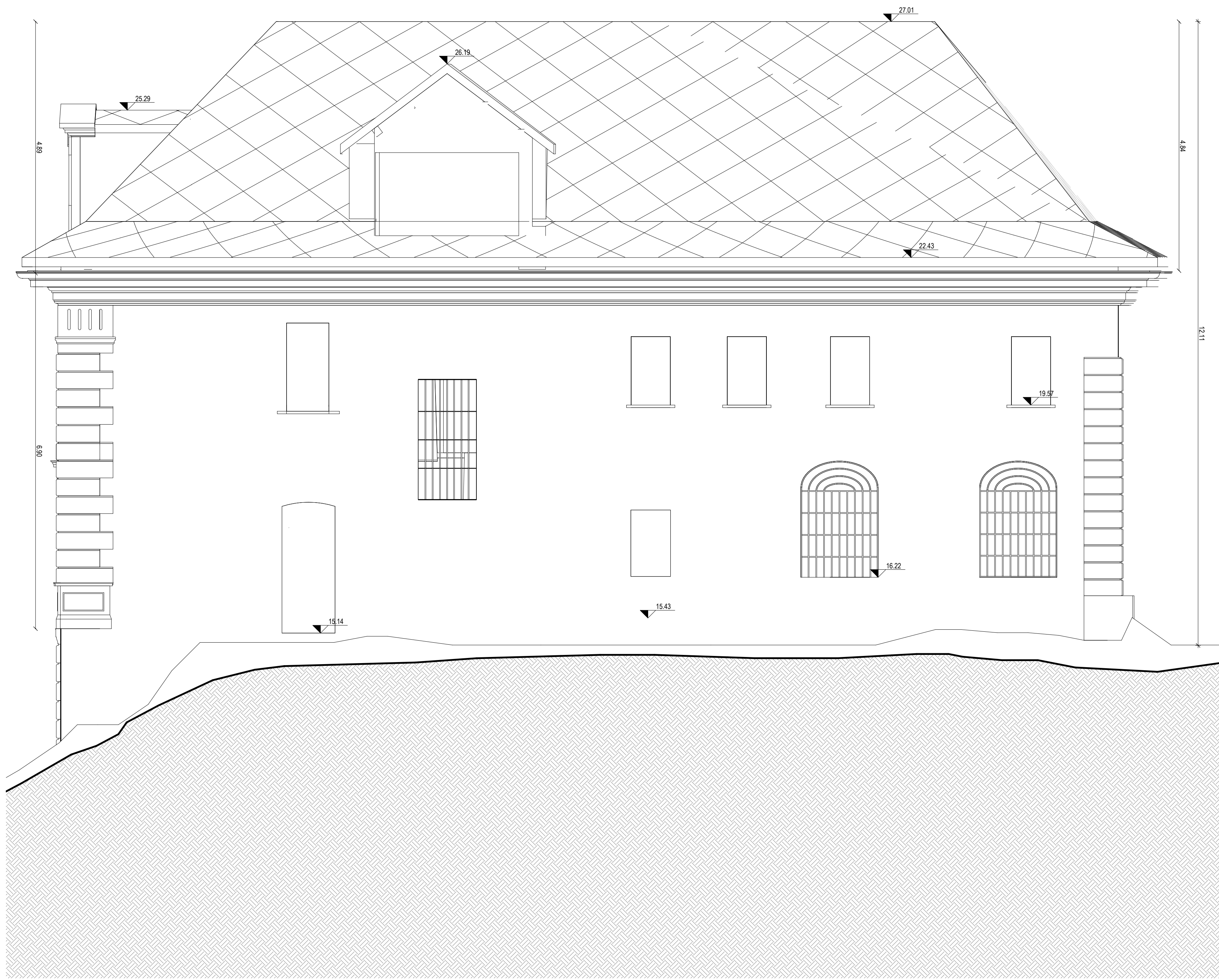
1 prospetto est - rilievo
