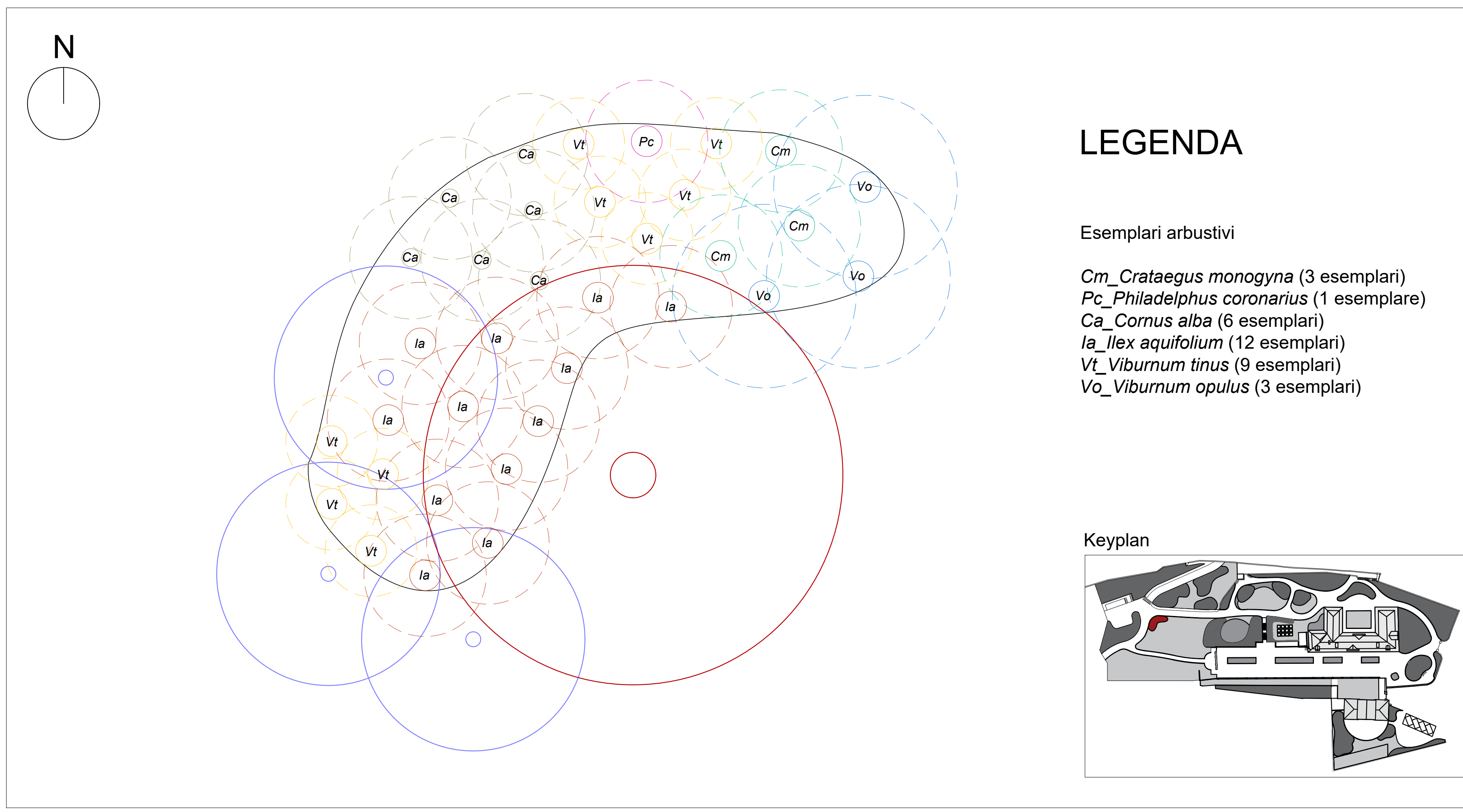
AIUOLA 1bis_F 1:50
