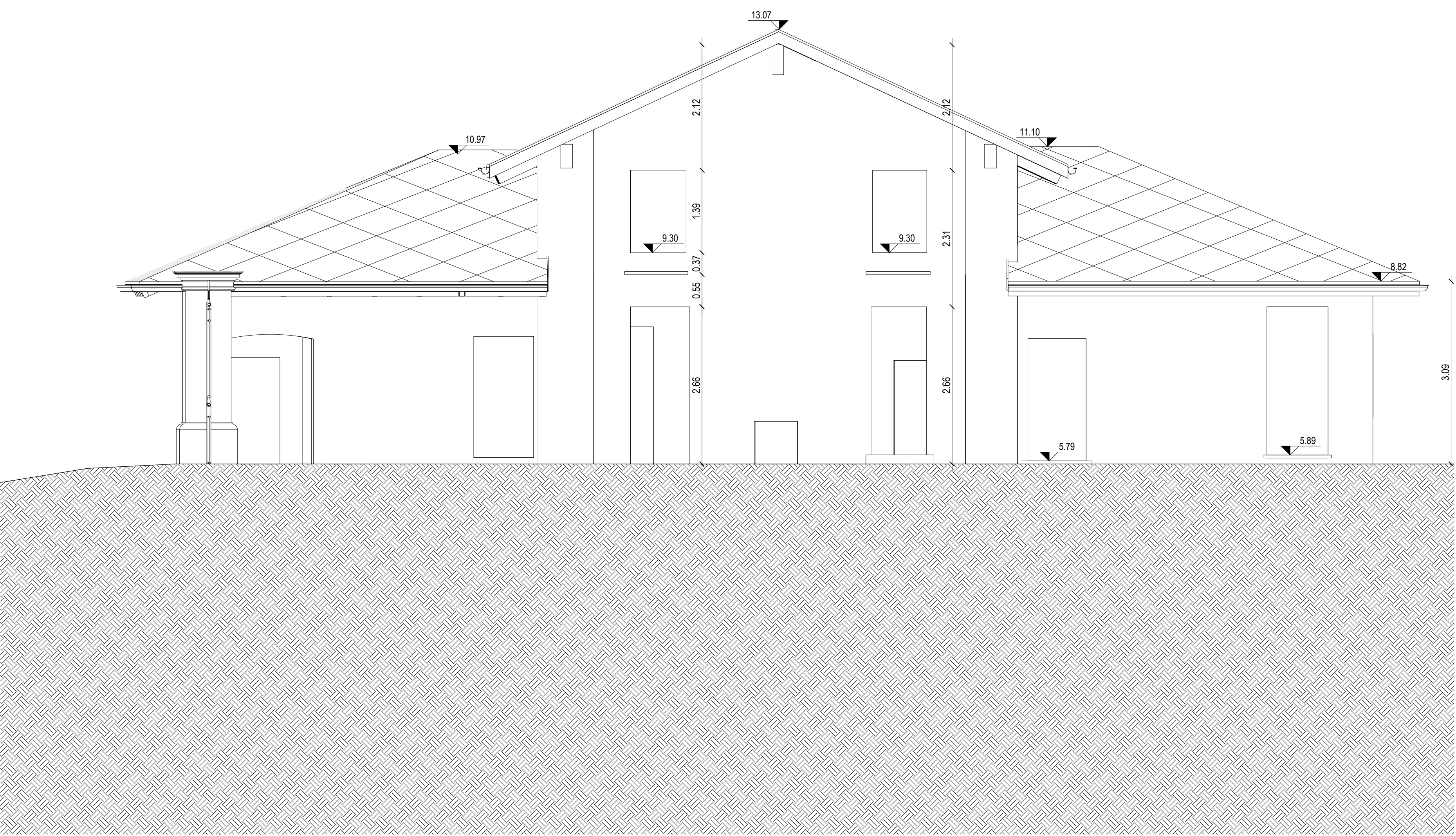
4 prospetto NORD - rilievo
