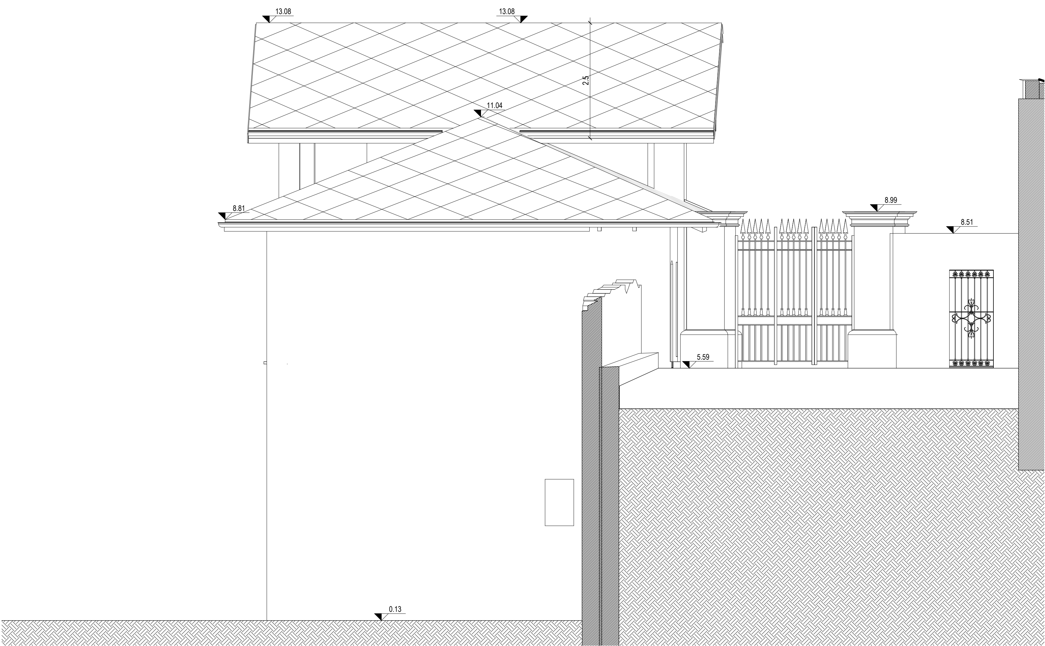
3 prospetto EST - rilievo
