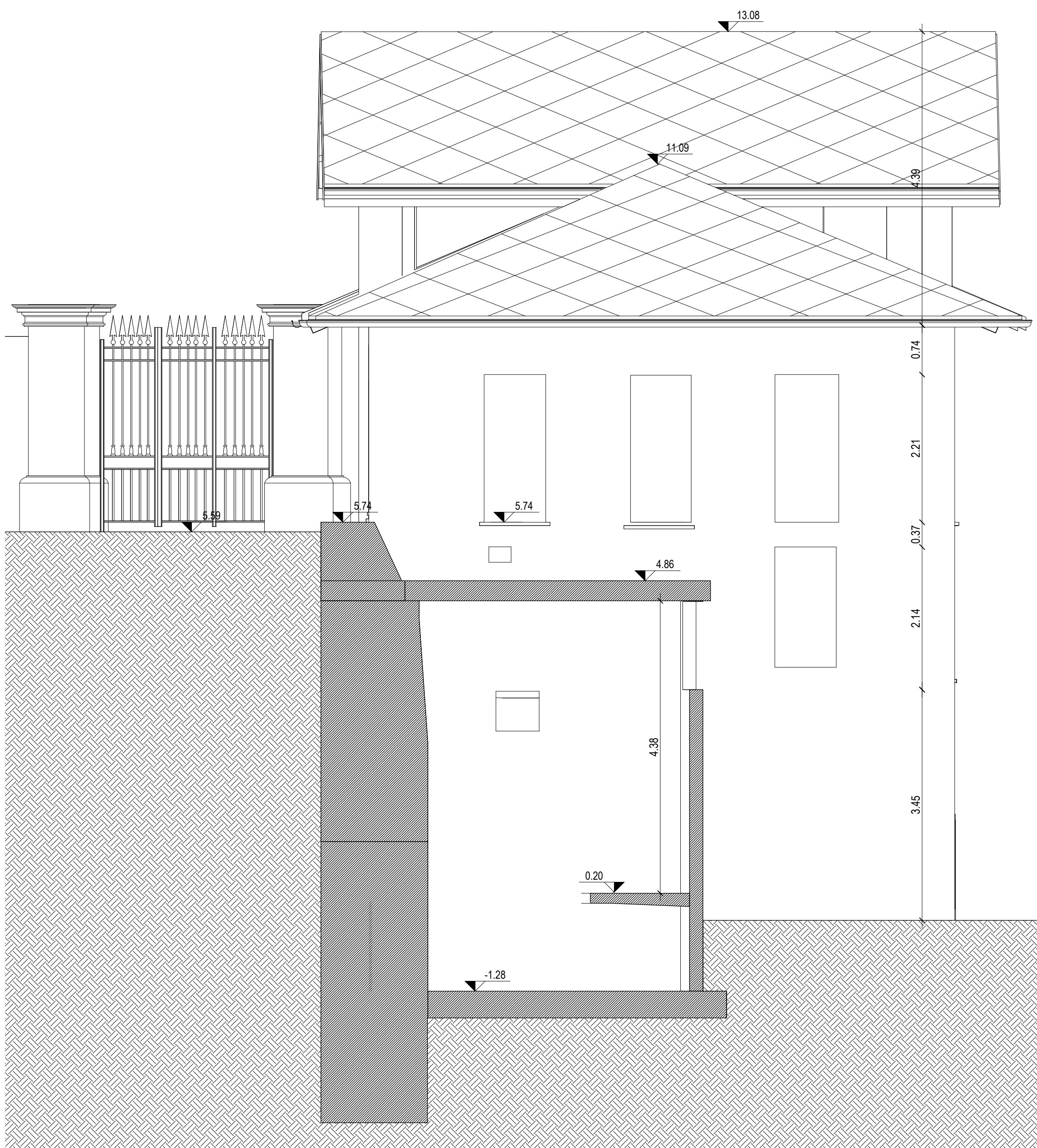
1 prospetto OVEST - rilievo
