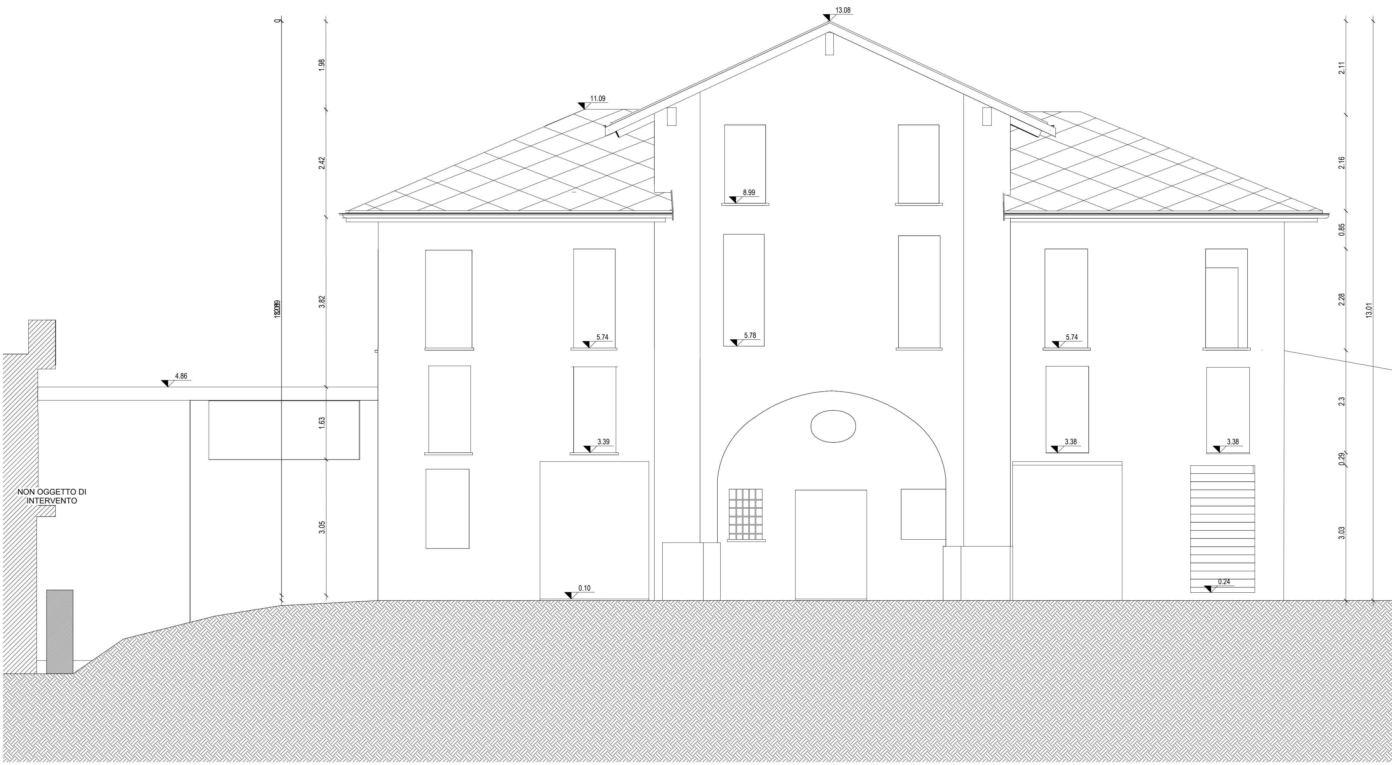
2 prospetto SUD - rilievo
