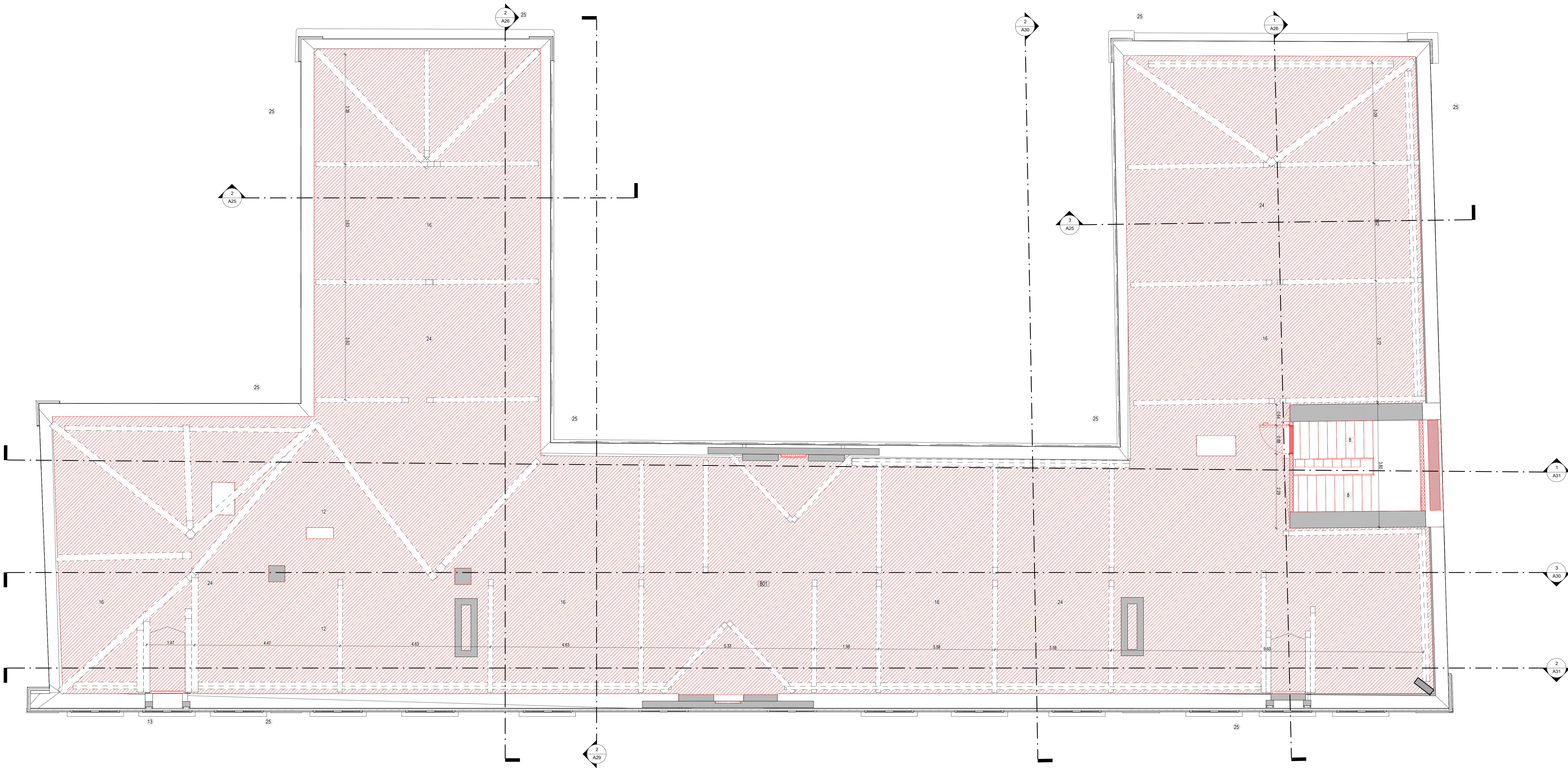
0 piano sottotetto - costruzioni
