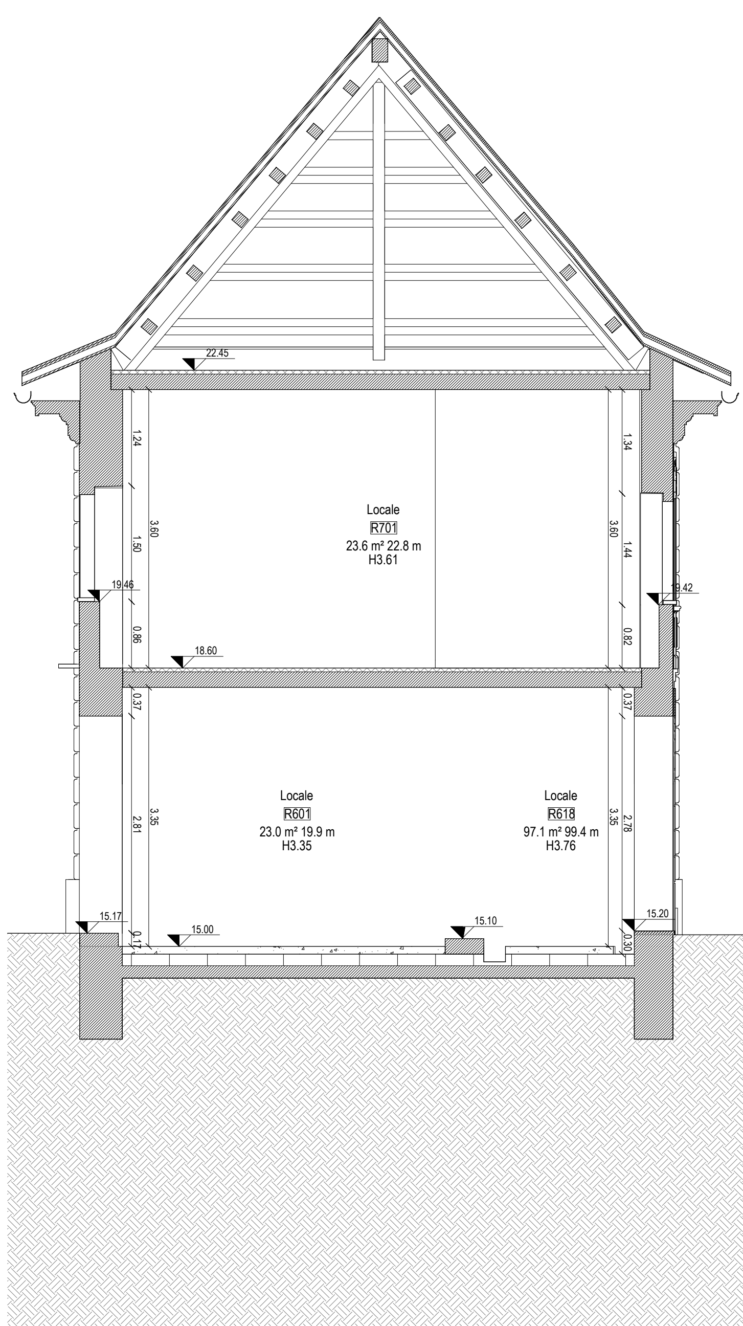
② sezione BB - rilievo
