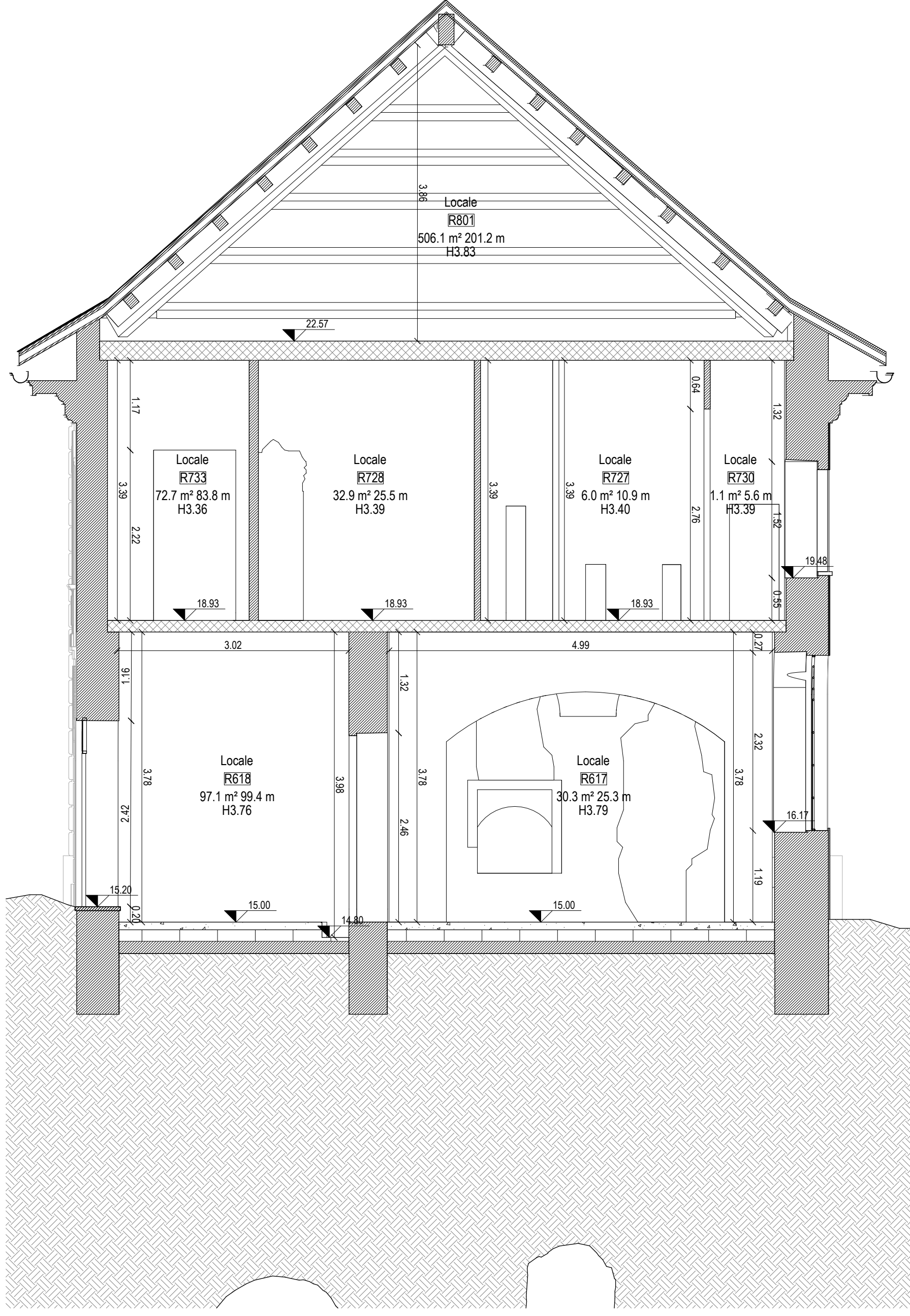
③ sezione CC - rilievo
