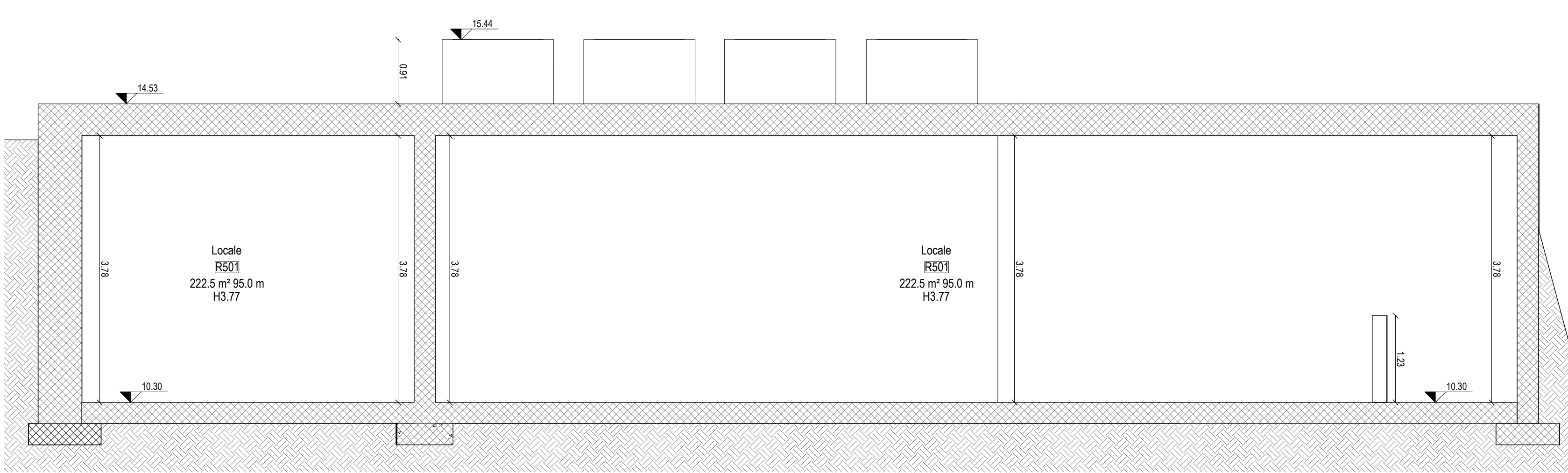
① sezione AA - rilievo
