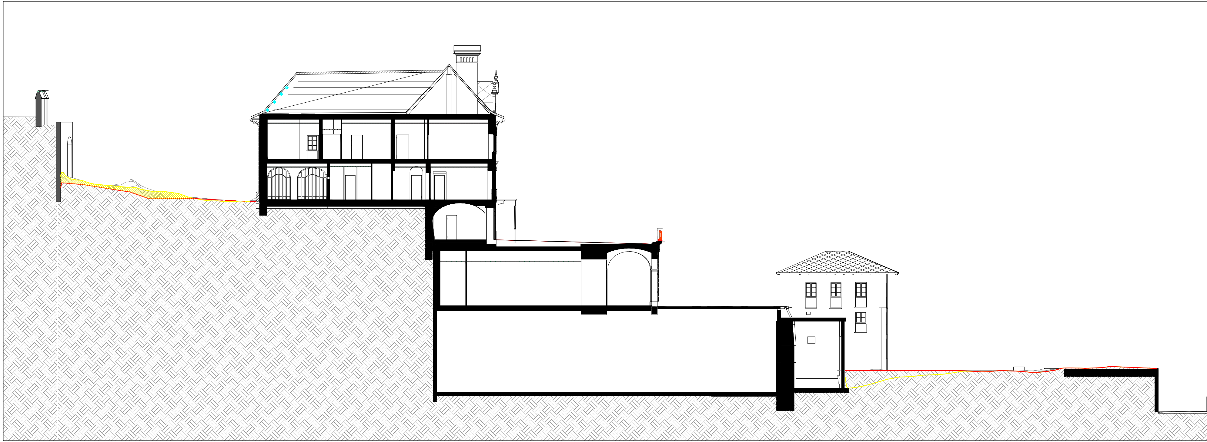
4 Sezione CC - comparativa
