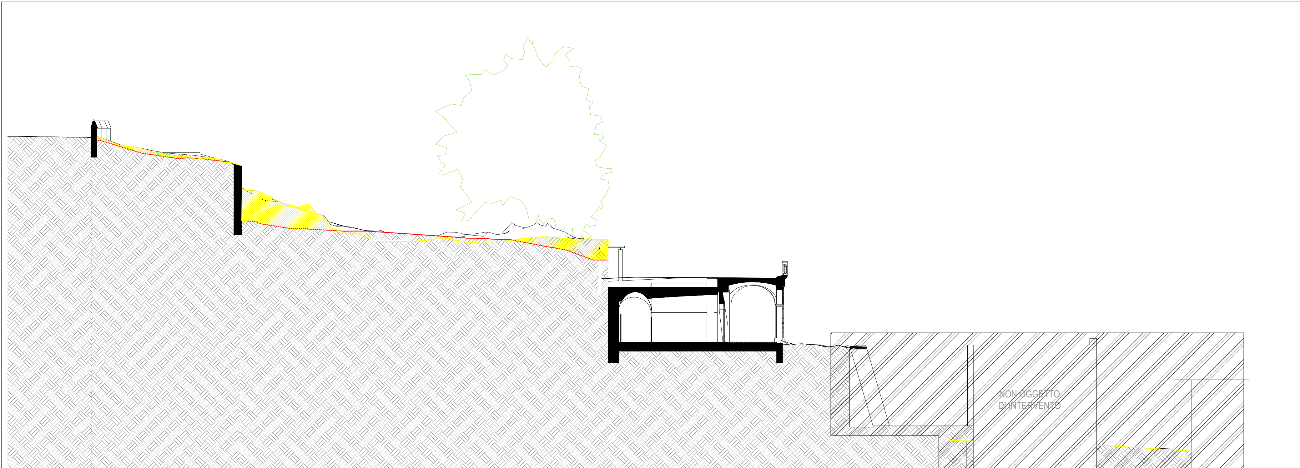
1 Sezione FF - comparativa
