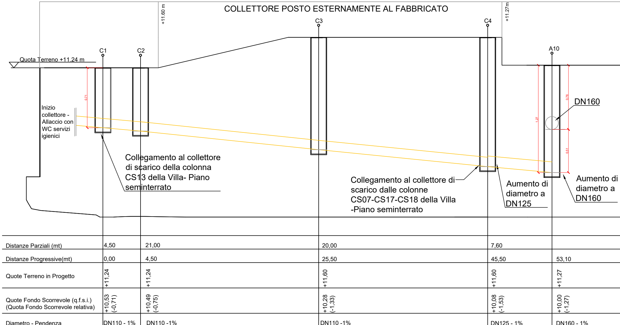
PROFILO SCARICO ACQUE NERE - TRATTO C1-A10
