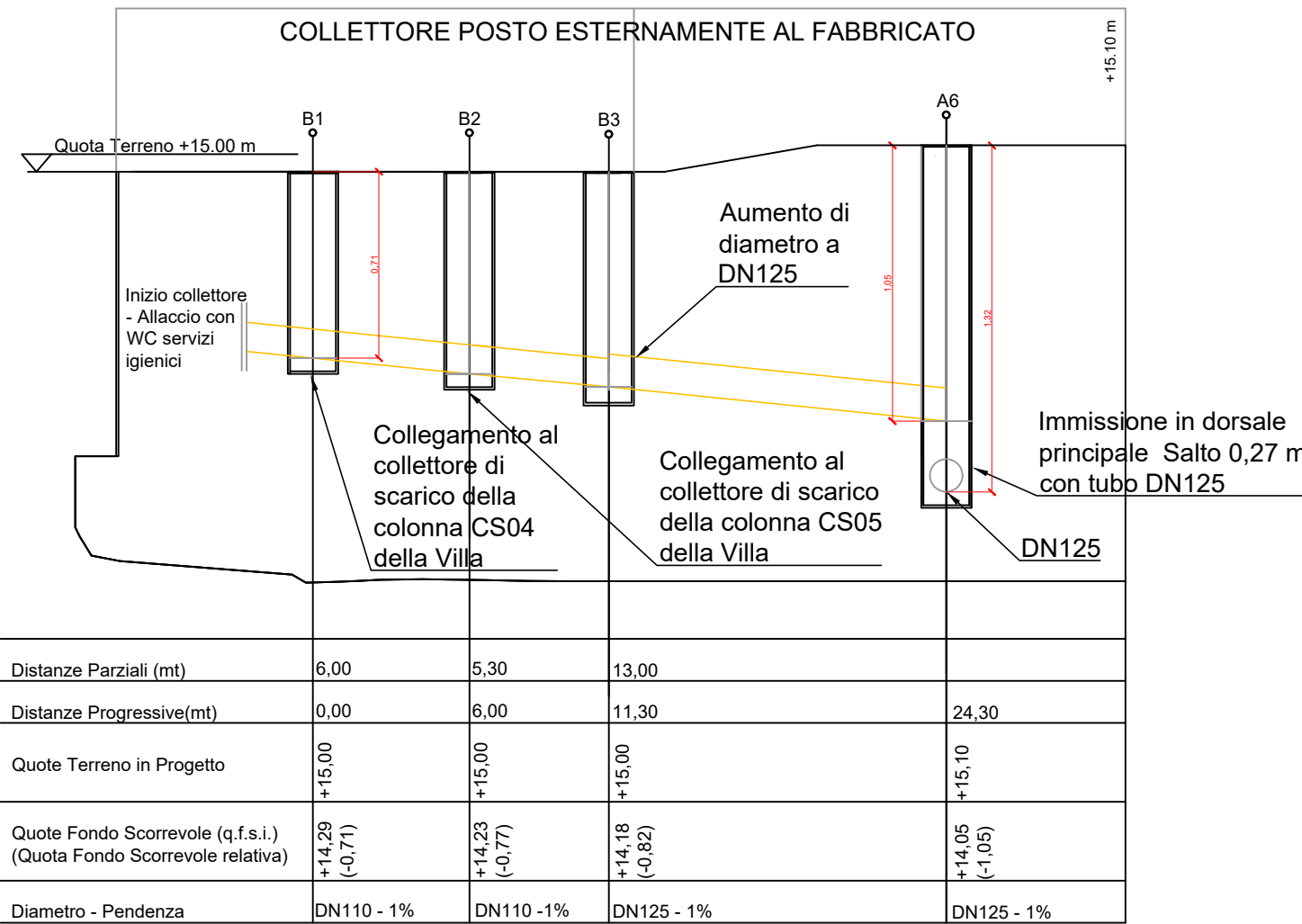
PROFILO SCARICO ACQUE NERE - TRATTO B1-A6
