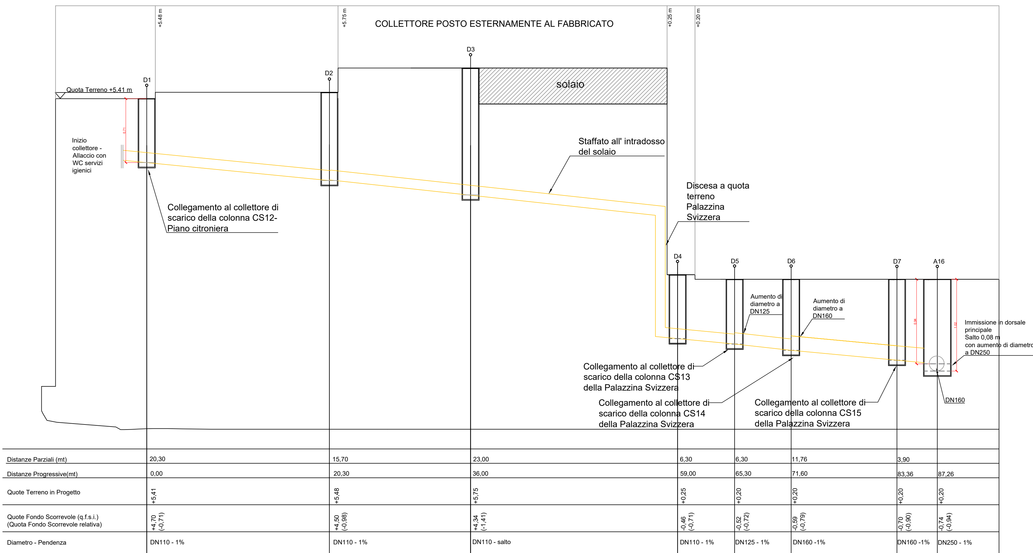
PROFILO SCARICO ACQUE NERE - TRATTO D1-A16
