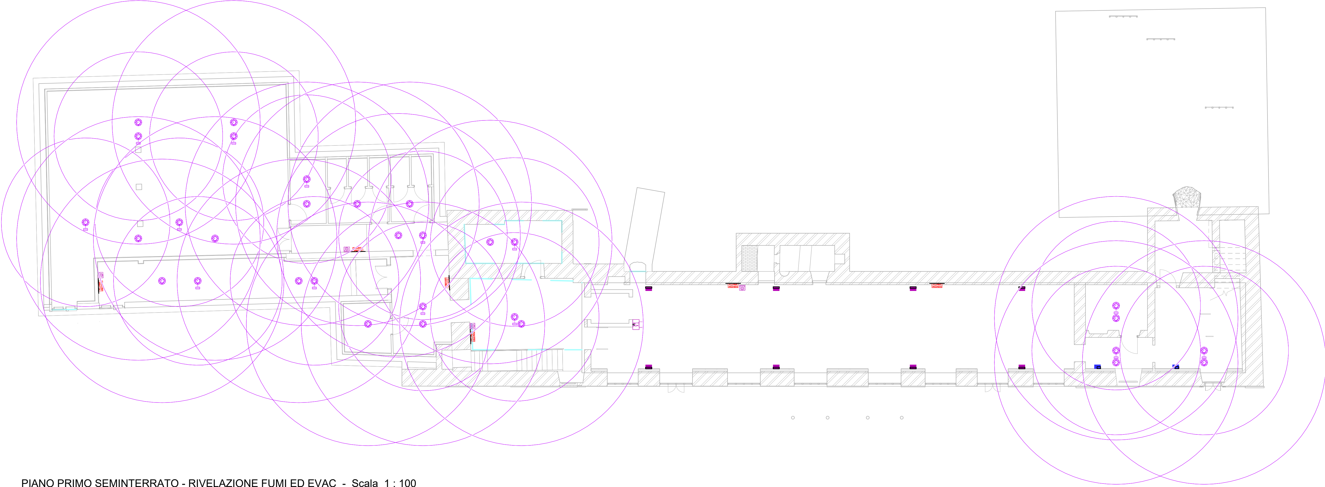
PIANO PRIMO SEMINTERRATO - RIVELAZIONE FUMI ED EVAC - Scala 1 : 100
