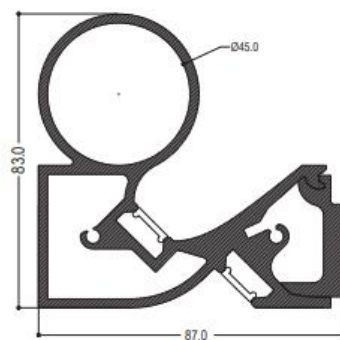
SEZIONE/SECTION
