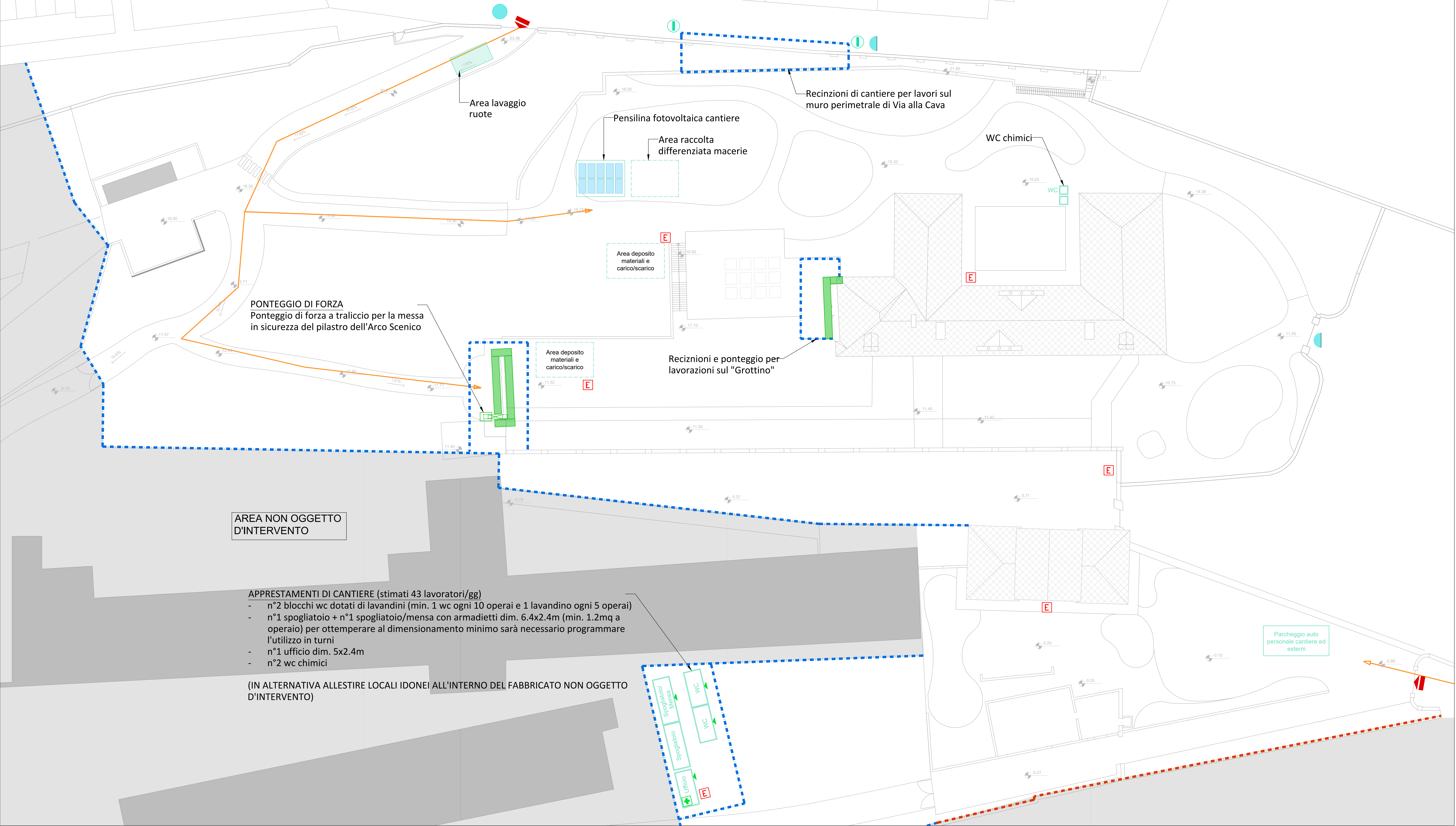
PLANIMETRIA - SISTEMAZIONI ESTERNE - SCALA 1:200
